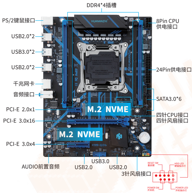
图1-1 X99-QD4主板图解
