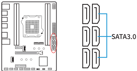
图2 -11 SATA接口
